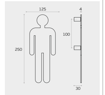
IN.26.416.P Silhuetas para casa de banho com fixação oculta por parafuso / Bathroom indicators with concealed fixing at the wall / Indicadores de toilette con sujeción oculta por tornillos.
