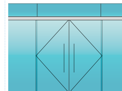
IN.15.707.4000 IN.15.707.6000 Carril para suspensão no vidro fixo / Track for suspension on fixed glass / Carril para sujetar al cristal fijo.
