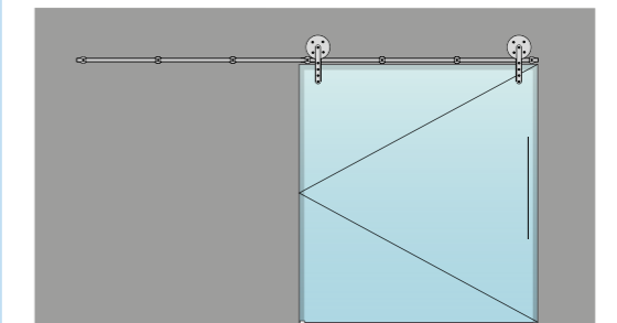
(A) FIXAÇÃO À PAREDE / FIXED AT WALL / FIJADO A PARED
