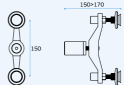
IN.82.005 Suporte para vidro com acessórios / Glass connector with accessories / Soporte para cristal con accesorios.
