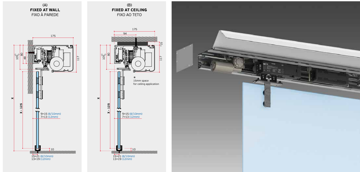
(B) FIXED AT CEILING / FIXO AO TETO
