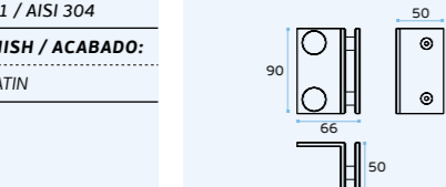
IN.05.305 Suporte de parede-vidro / Wall to glass support / Soporte pared-cristal.
