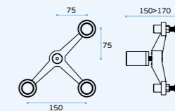
IN.82.006 Suporte para vidro com acessórios / Glass connector with accessories / Soporte para cristal con accesorios.
