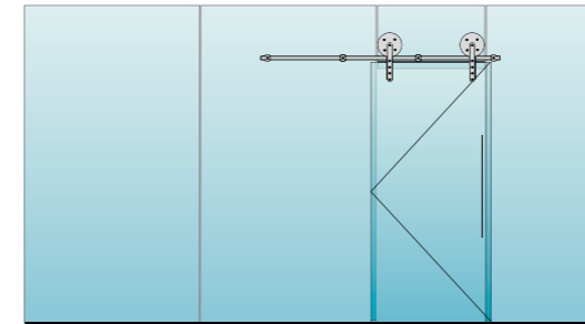
(B) FIXED AT GLASS / FIXO NO VIDRO / FIJO EN CRISTAL
